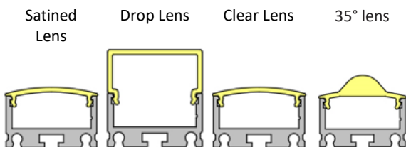
XT02 + XT99-SL XT02 + XT99-DL XT02 + XT99-CL XT02 + XT99-CL35
